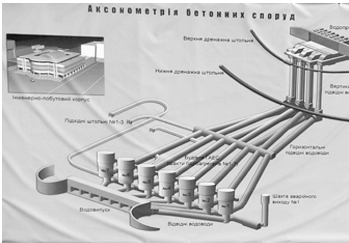
Схема ГАЕС.
